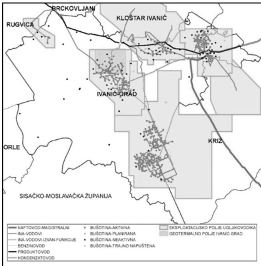
Slika 17: Energetska infrastruktura u vlasništvu Ina d.d. na području Grada Ivanić-Grad Izvor: INA d.d., 2021. Obrada: Zavod za prostorno uređenje Zagrebačke županije, 2021.
